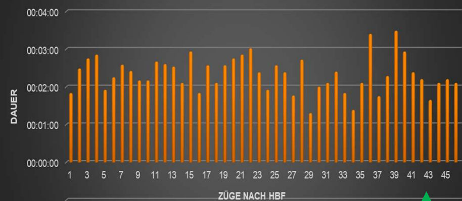
Dauer Schließzeit bei "Zug fährt zum HBF"
